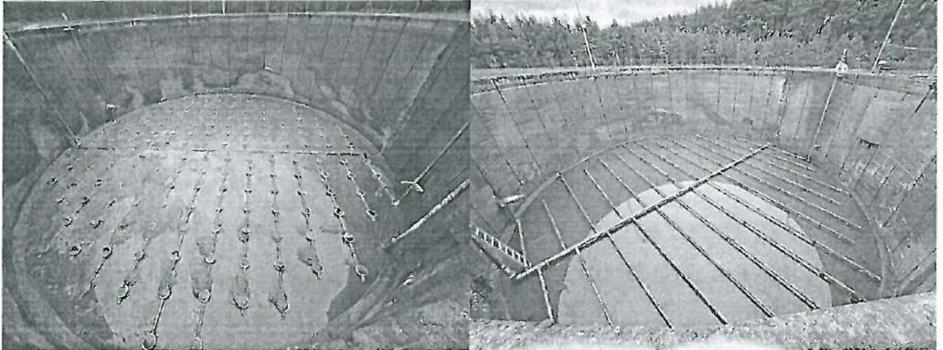
38 pav. Varėnos miesto buitinių nuotekų valymo įrenginių aerotanko tvarkymas
